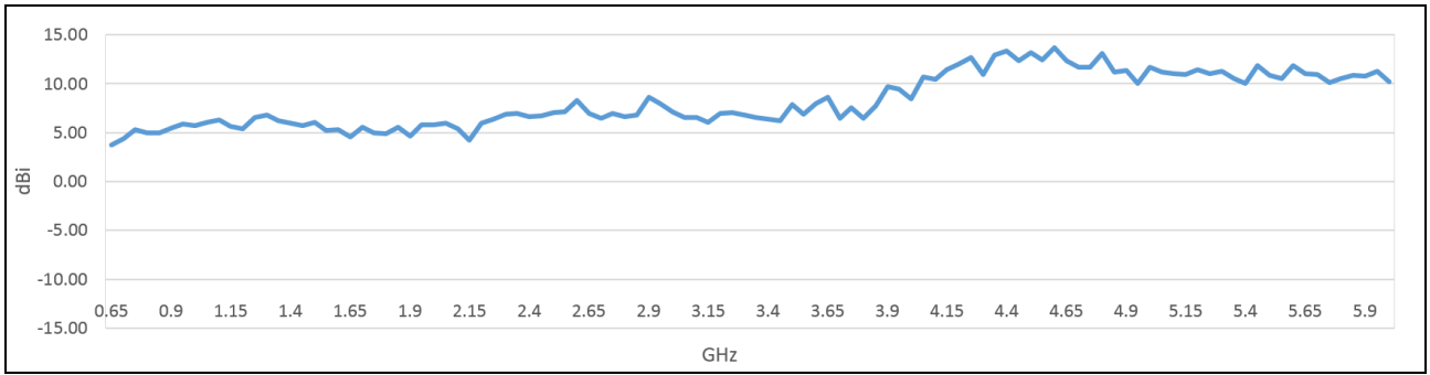
方向图Phi=0
